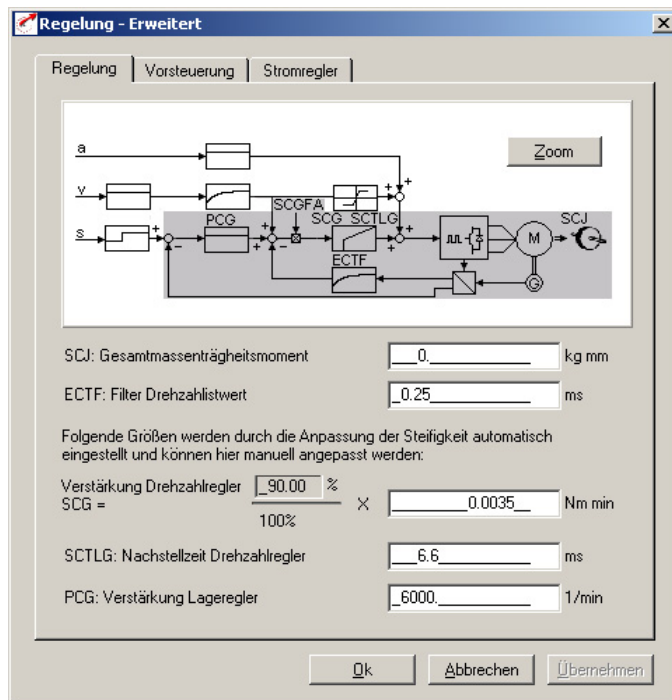
Bild 5.39 Register Regelung erweitert
