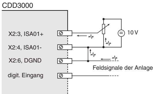
Bild 2.6 Störbeeinflussung des analogen Eingangs
