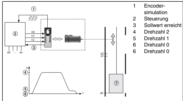
Bild 4.16 Beispiel eines Hubantriebs mit Eilgang-Schleichgang-Positionierung.
