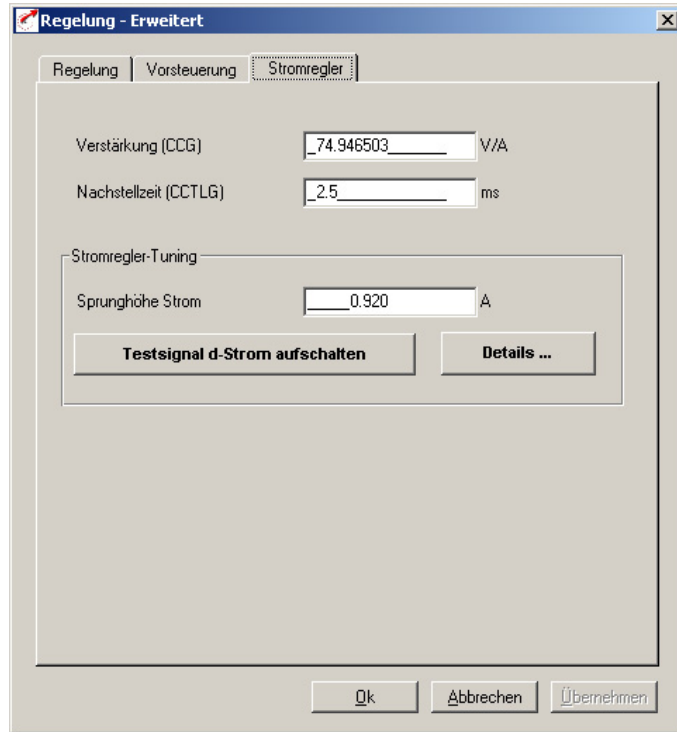
Bild 5.42 Stromregler
