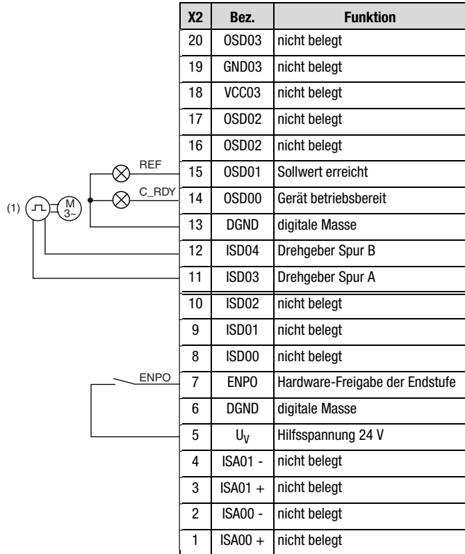
Bild 4.26 Klemmenbelegung bei Drehzahlregelung, Impulseingang, Steuern über Feldbus
