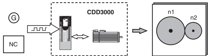
Bild 4.21 Drehzahlregelung über Impulseingang
