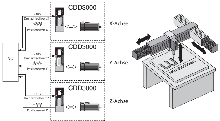
Bild 4.7 Beispiel einer 3-Achsen-Bahnsteuerung
