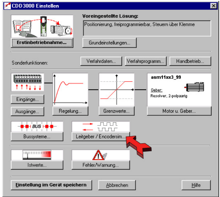
Bild 5.74 Bedienmaske Leitgeber / Encodersimulation
