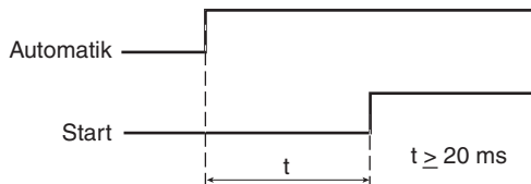
Bild 5.13 Timing AUTO
