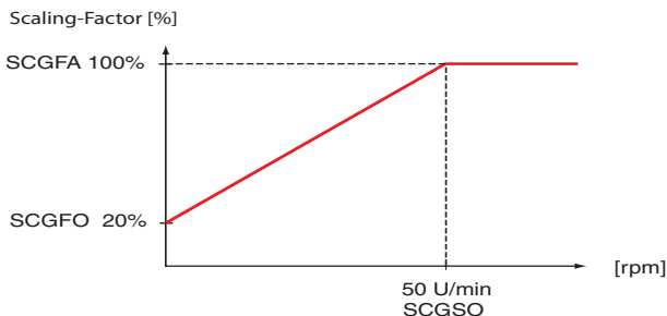
Bild 5.40 Reduktion der Drehzahlreglerverstärkung bei kleinen Drehzahlen
