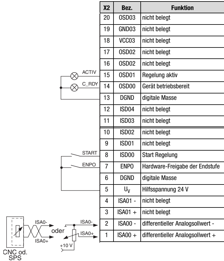
Bild 4.14 Klemmenbelegung bei Drehzahlregelung, \pm 10\text{ V} Sollwert, Steuern über Klemme
