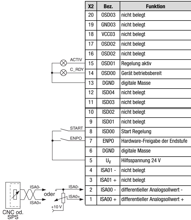
Bild 4.6 Klemmenbelegung bei Drehmomentregelung, ± 10 V Sollwert, Steuern über Klemme
