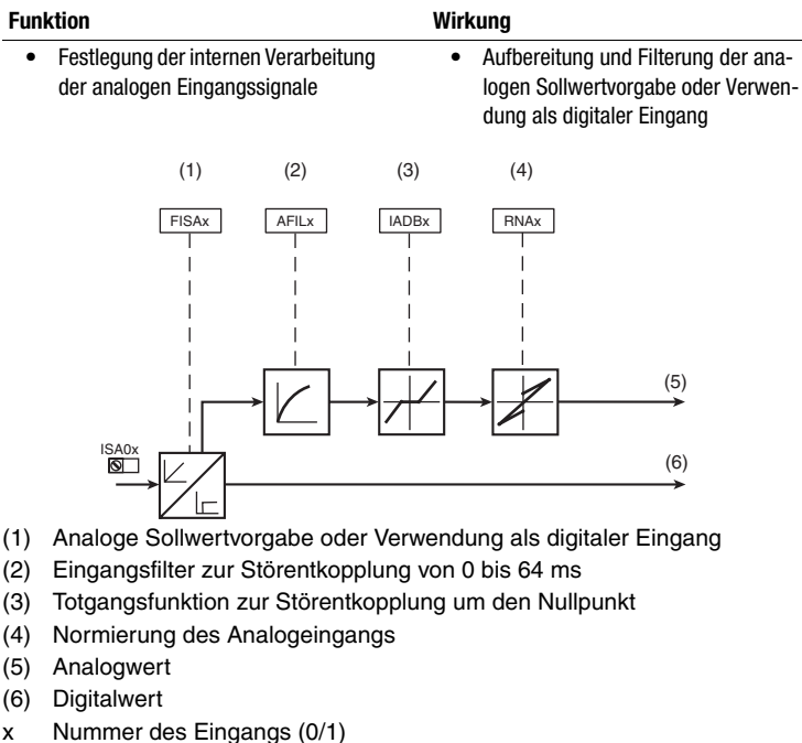
Bild 5.2 Funktionsblock zur Anpassung der analogen Eingänge
