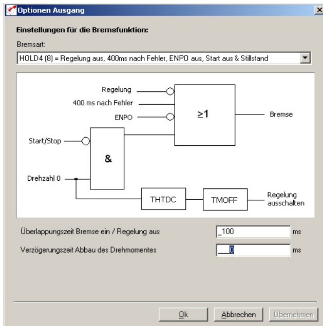
Bild 5.19 Einstellung der Bremsfunktion
