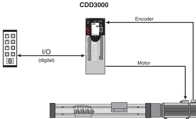
Bild 4.54 Prinzipieller Aufbau eines Positioniersystems
