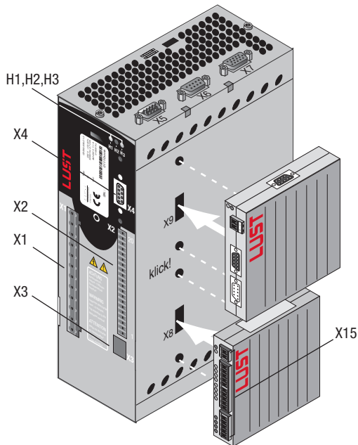
Bild 2.1 Lageplan CDD3000
