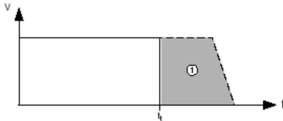
Bild 4.84 Triggerbezogener Vorschub. (1) Markensensor
