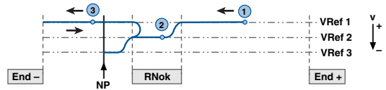
Bild 4.46 Referenzfahrttyp 1. Der Referenznocken befindet sich zwischen den beiden Hardware-Endschaltern. Der auszuwertende Nullimpuls soll der erste nach Verlassen des Nockens in negativer Richtung sein.
