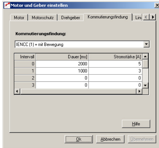
Bild 5.58 Register Kommütierungsfindung mit Bewegung
