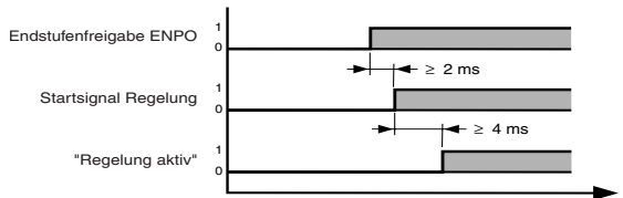
Bild 4.78 Timing der Ansteuerung „START-Regelung“
