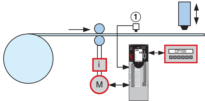
Bild 4.84 Triggerbezogener Vorschub. (1) Markensensor
