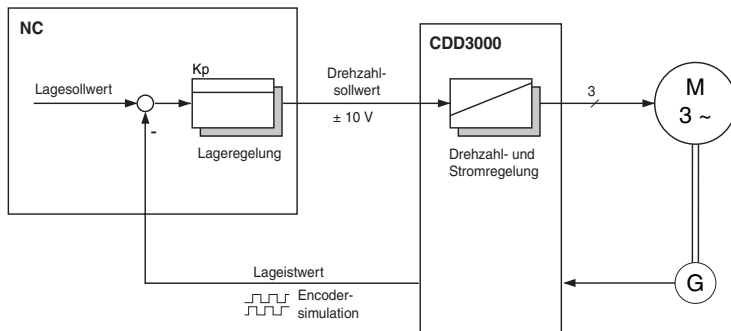
Bild 4.8 Prinzipdarstellung der Regelstruktur
