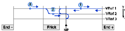
Bild 4.63 Referenzfahrttyp 2: Der Referenznocken befindet sich zwischen den beiden Hardware-Endschaltern, Auswertung des erster Nullimpulses nach Verlassen des Nockens in positiver Richtung siehe Tabelle 4.36
