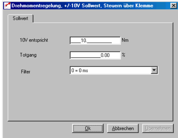
Bild 4.5 Register Sollwert
