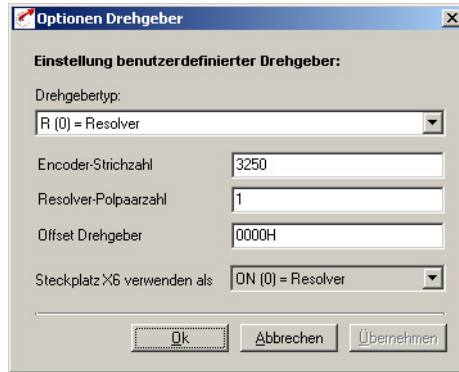
Bild 5.56 Optionen Drehgeber
