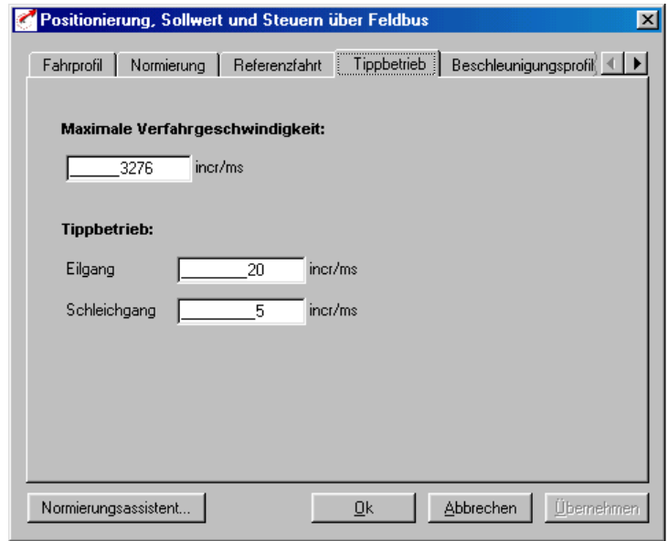
Bild 4.36 Register Tippbetrieb
