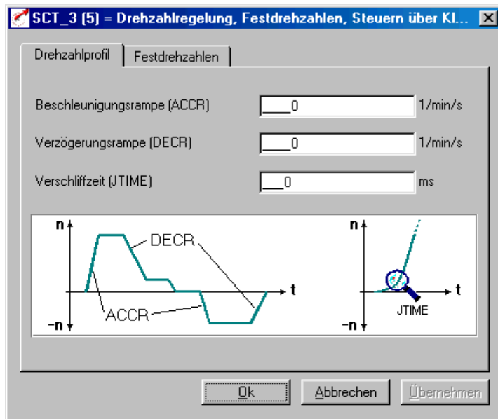
Bild 4.17 Register Drehzahlprofil
