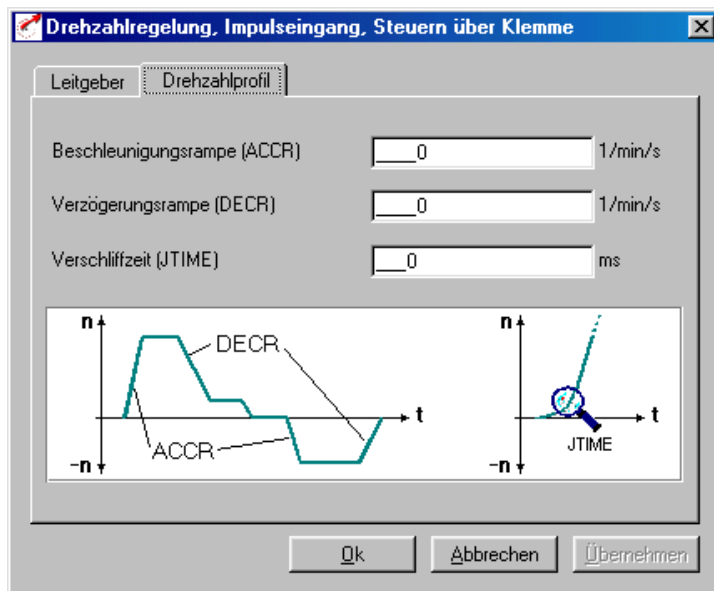
Bild 4.24 Register Drehzahlprofil
