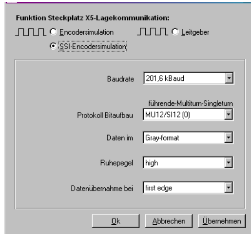
Bild 5.81 Register SSI-Encodersimulation
