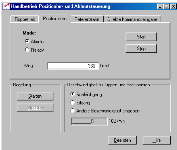
Bild 4.74 Register Positionieren
