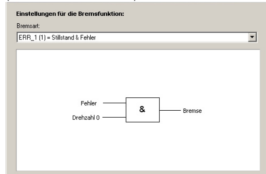
Bild 5.22 ERR_1
