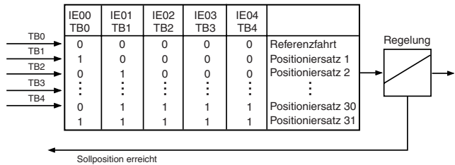
Bild 4.41 Sollwertaufbereitung
