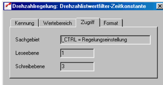
Bild 3.5 Zugriff
