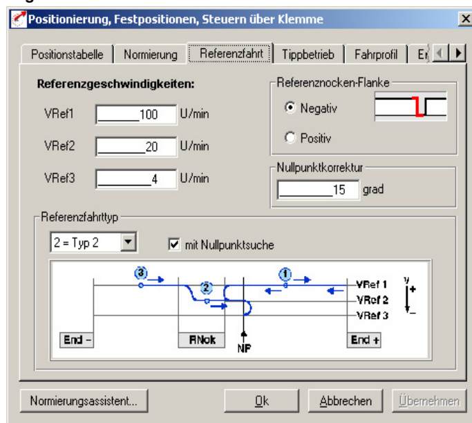
Bild 4.44 Register Referenzfahrt
