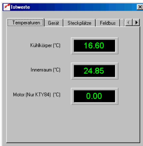
Bild 5.63 Register Temperaturen
