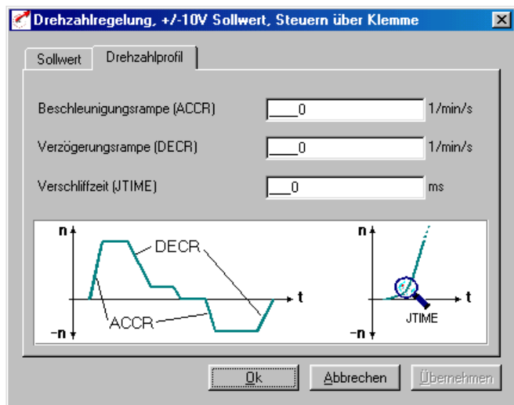
Bild 4.13 Parametermaske Drehzahlprofil
