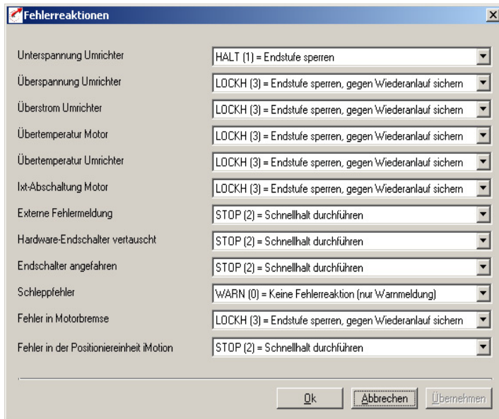
Bild 5.68 Fehlerreaktionen
