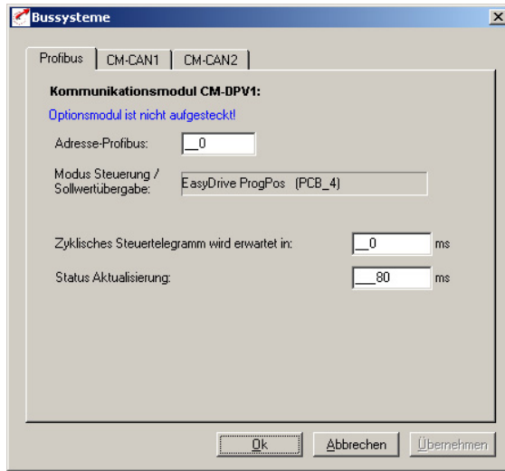
Bild 5.70 Register PROFIBUS
