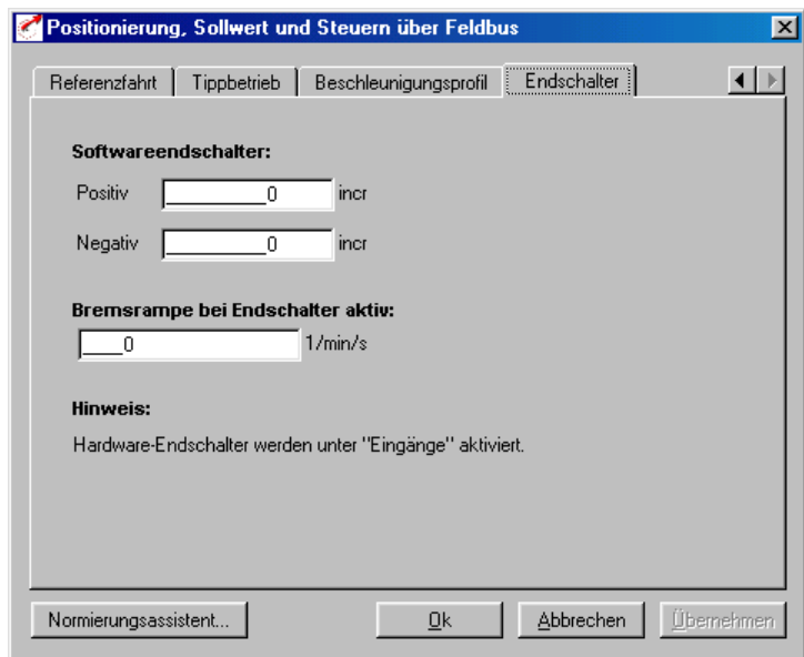
Bild 4.38 Register Endschalter
