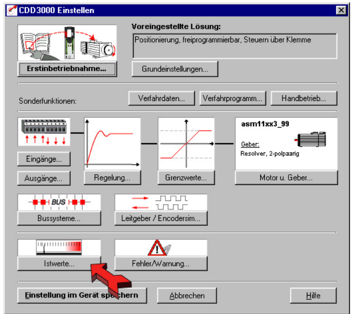
Bild 5.62 Bedienmaske Istwerte
