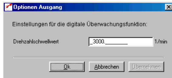
Bild 5.31 Drehzahlschwellwert
