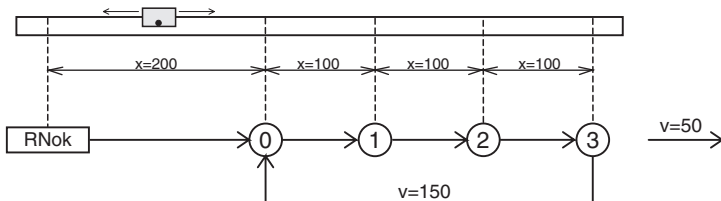
Bild 4.89 Positionen anfahren
