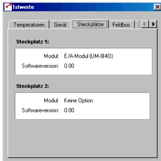
Bild 5.65 Register Steckplätze
