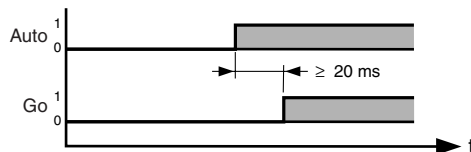
Bild 4.79 Timing der Ansteuerung „Go“
