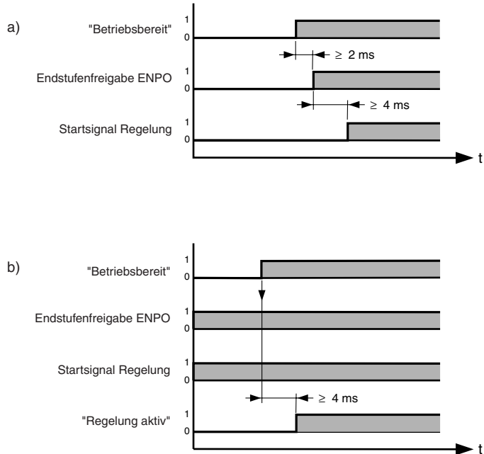
Bild 5.10 (Einschaltvorgang a) ohne Auto-Start und b) mit Auto Start
