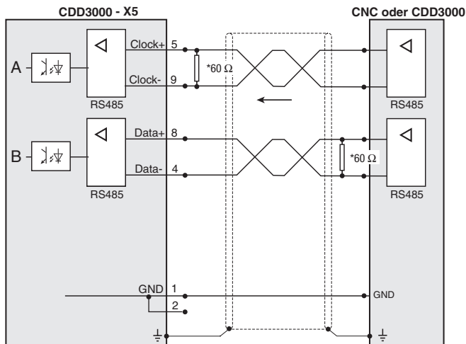
Bild 5.82 Anschluß- und Signalbeschreibung der SSI-Encodersimulation
