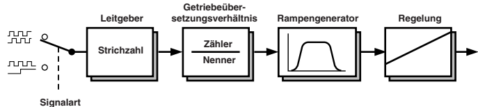
Bild 4.22 Struktur der Sollwertaufbereitung
