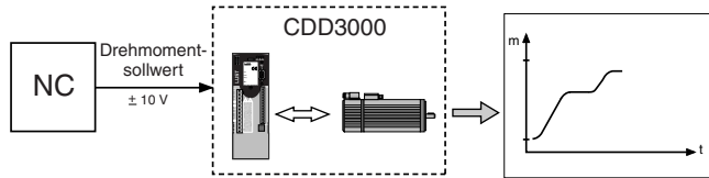
Bild 4.4 Drehmomentregelung mit \pm 10 V Sollwertvorgabe
