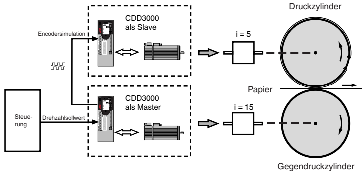
Bild 4.83 Beispiel einer Druckmaschine
