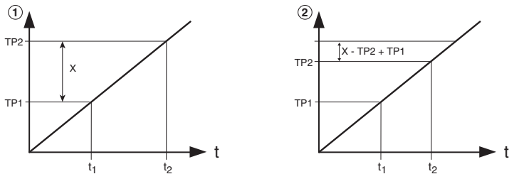
Bild 4.88 (1): Optimaler Eintreffzeitpunkt für beide TouchProbes. (2): TouchProbe 2 kommt zu früh.
