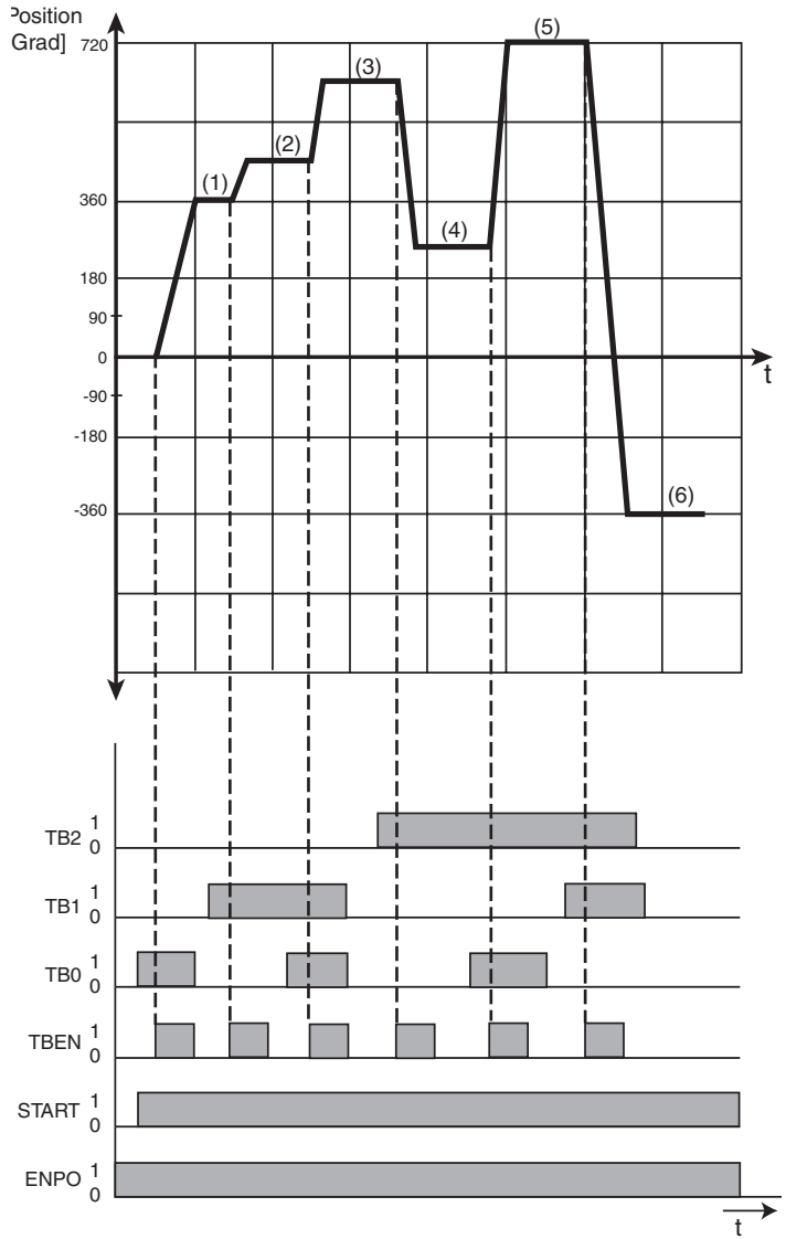
Bild 4.53 Beispiel zu Positionierung mit Festpositionen
