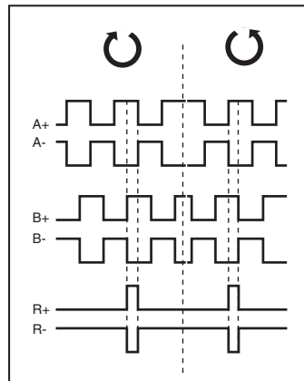
Bild 5.77 Signale der Encodersimulation bei Blick auf die Motorwelle (links bei Rechtslauf des Motors)
