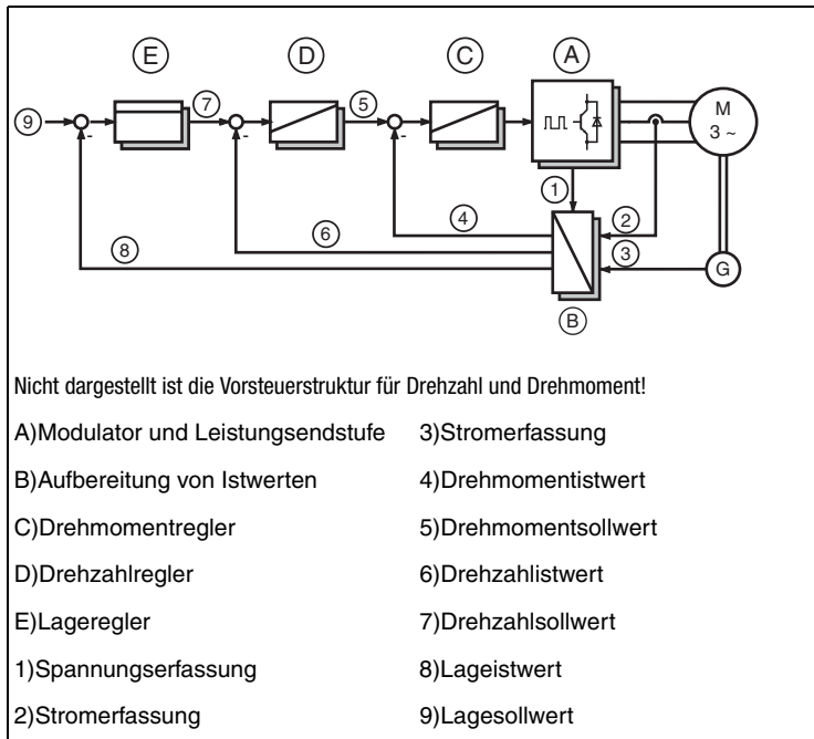
Bild 5.36 Regelungsstruktur
