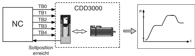
Bild 4.40 Positionierung mit Festposition, Steuern über Klemme
