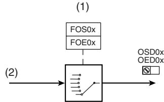
Bild 5.17 Funktionsblock zur Anpassung der digitalen Ausgänge
