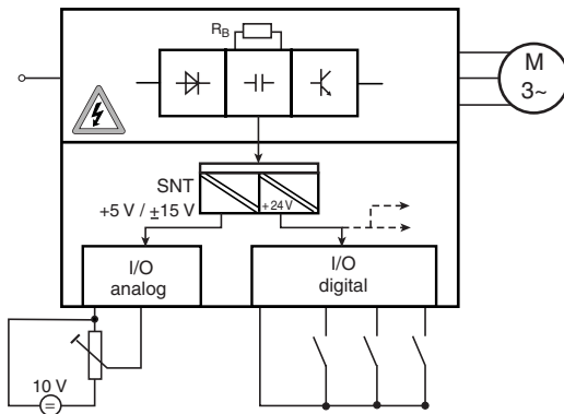
Bild 2.4 Spannungsversorgung der E/As
