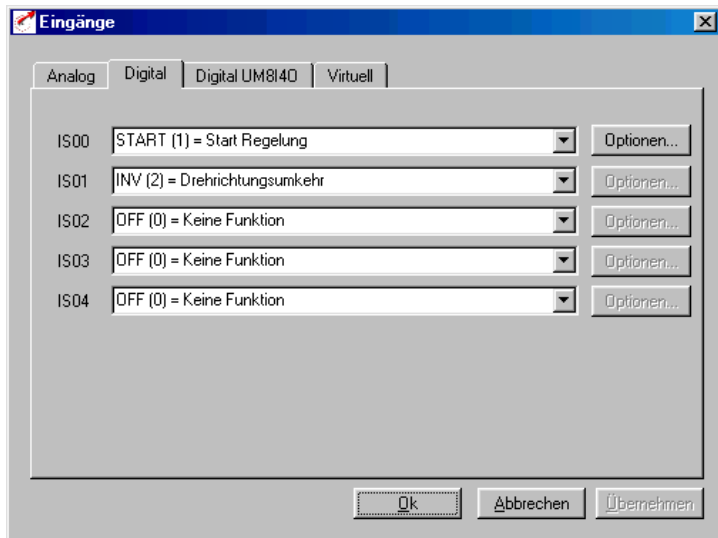
Bild 5.8 Register Digitale Eingänge
