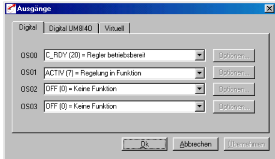
Bild 5.18 Register Digitale Ausgänge
