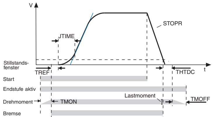
Bild 5.20 Drehzahlprofil Bremsfunktion
