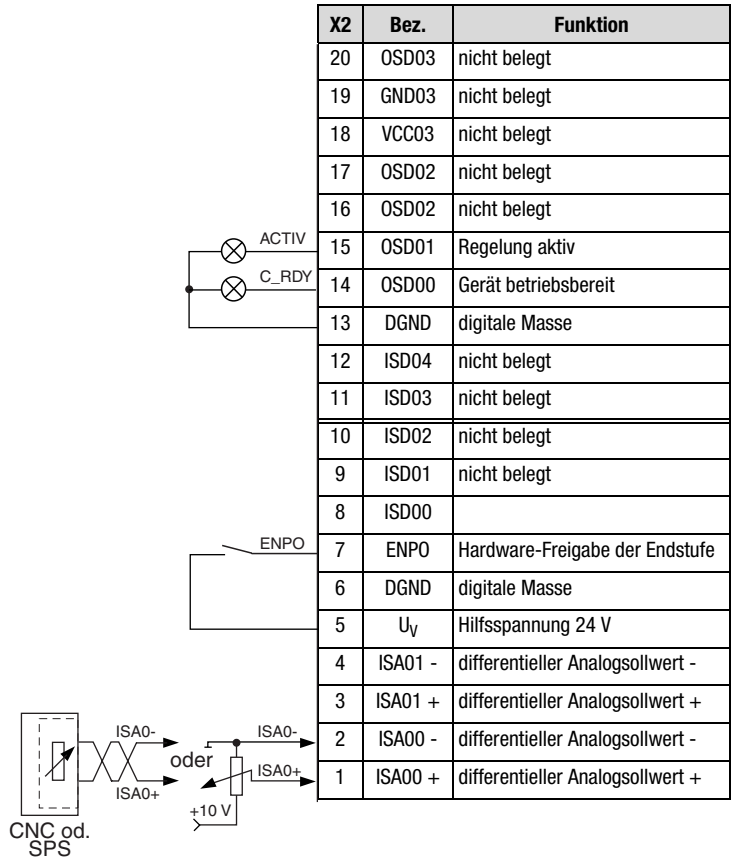
Bild 4.15 Klemmenbelegung bei Drehzahlregelung, \pm 10 V Sollwert, Steuern über Feldbus
