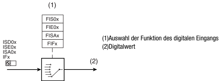
Bild 5.7 Funktionsblock zur Anpassung der digitalen Eingänge
