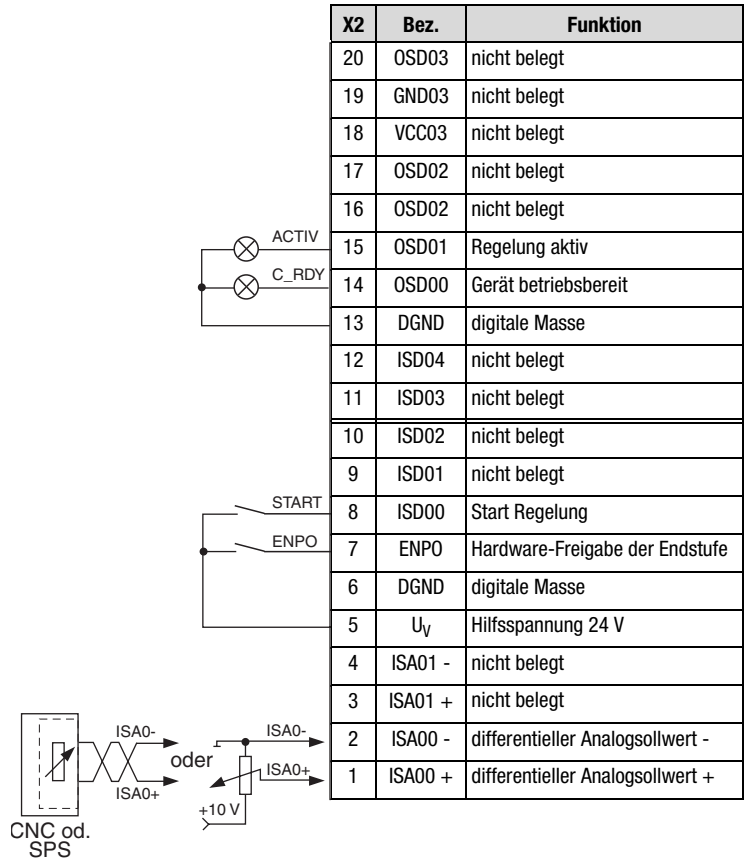
Bild 4.10 Klemmenbelegung bei Drehzahlregelung mit externer Lageregelung, Steuern über Klemme
