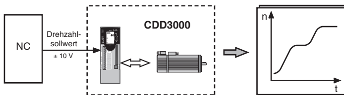
Bild 4.11 Drehzahlregelung mit \pm 10 V Sollwertvorgabe
