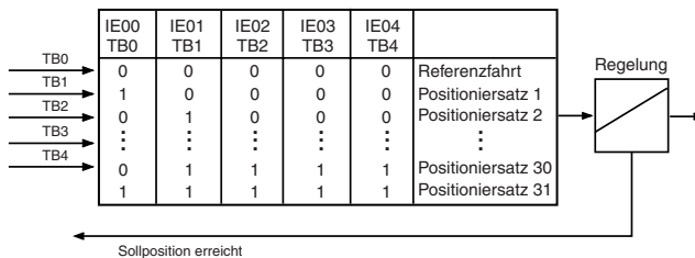
Bild 5.11 Sollwertaufbereitung: Positionierung, Festpositionen
