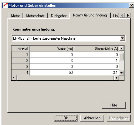
Bild 5.59 Register Kommütierungsfindung bei festgebremster Maschine
