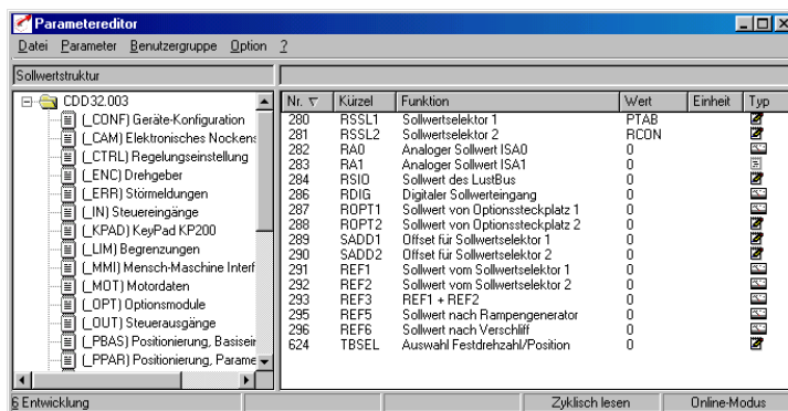
Bild 3.7 Parametereditor
