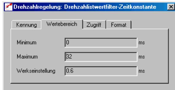
Bild 3.4 Wertebereich
