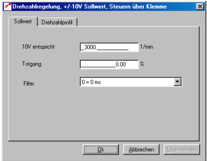
Bild 4.12 Register Sollwert
