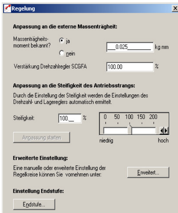
Bild 5.37 Register Regelung
