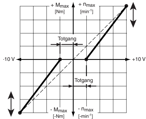
Bild 5.4 Konfigurationsmöglichkeiten ISA0
