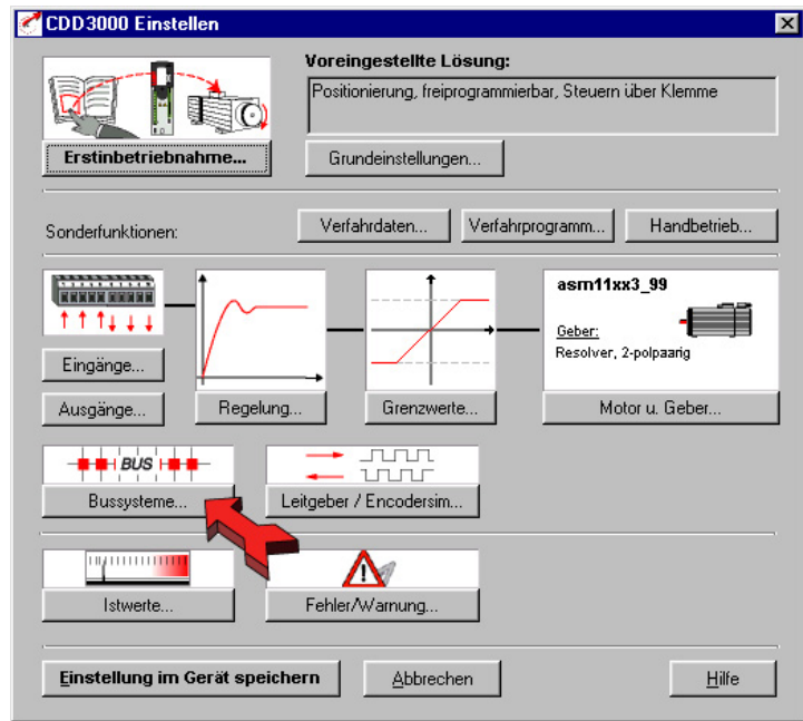
Bild 5.69 Bedienmaske Bussysteme
