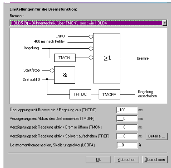
Bild 5.29 HOLD5
