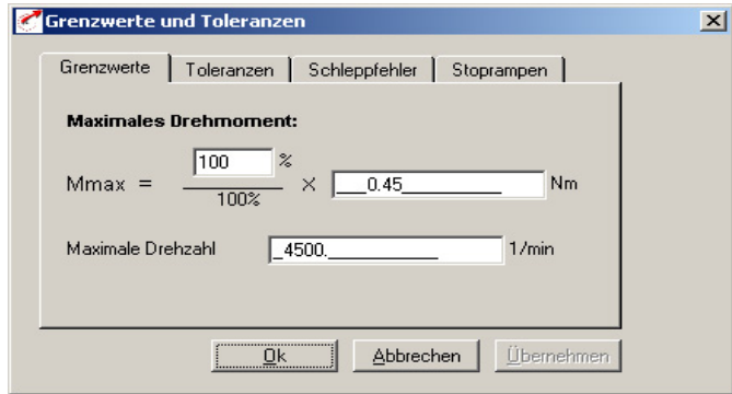
Bild 5.44 Register Grenzwerte
