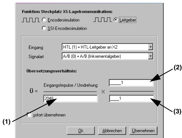
Bild 5.79 Register Leitgeber
