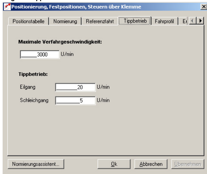
Bild 4.47 Register Tippbetrieb
