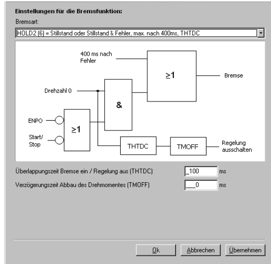
Bild 5.26 HOLD2
