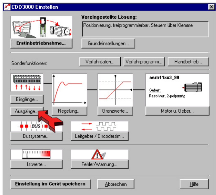
Bild 5.16 Bedienmaske Ausgänge
