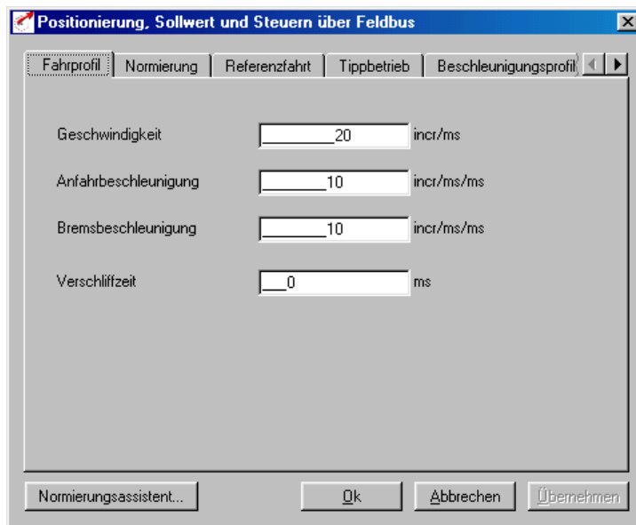
Bild 4.31 Register Fahrprofil
