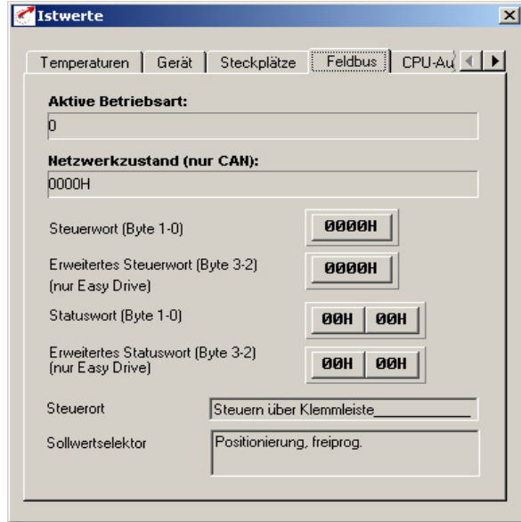
Bild 5.66 Register Feldbus
