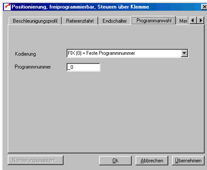
Bild 4.69 Register Programmanwahl
