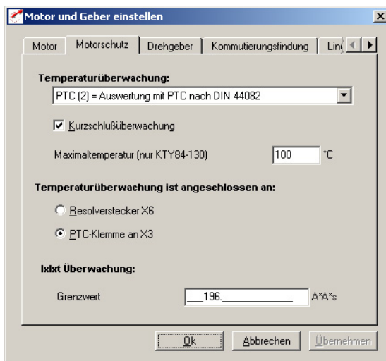
Bild 5.53 Register Motorschutz
