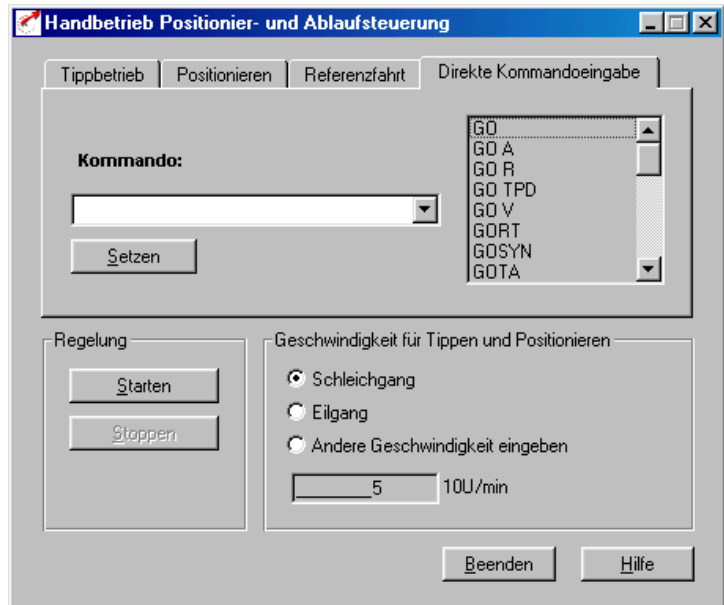
Bild 4.76 Register Kommando
